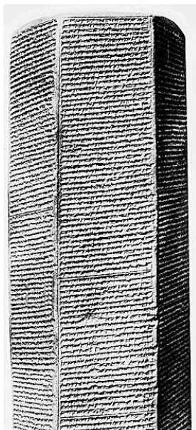
Призма Сеннахирима
